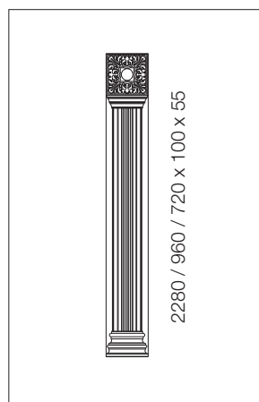
Oszlop
