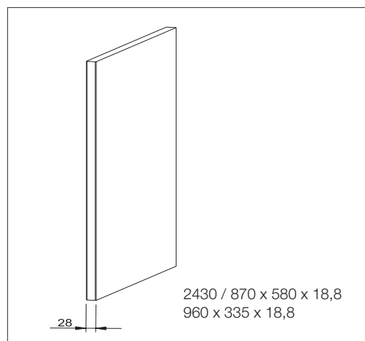
Végzáró panel
